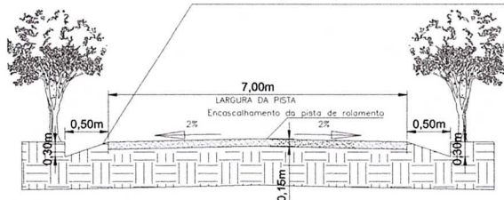
4 PERFIL TRANSVERSAL SEM ESCALA
